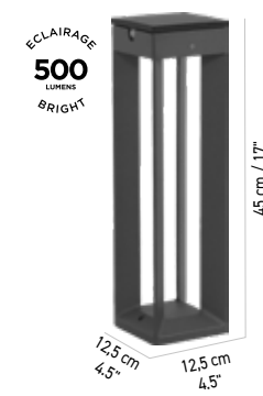
BORNE BLADE À FIXER BLADE PATHWAY LIGHT TO FIX
